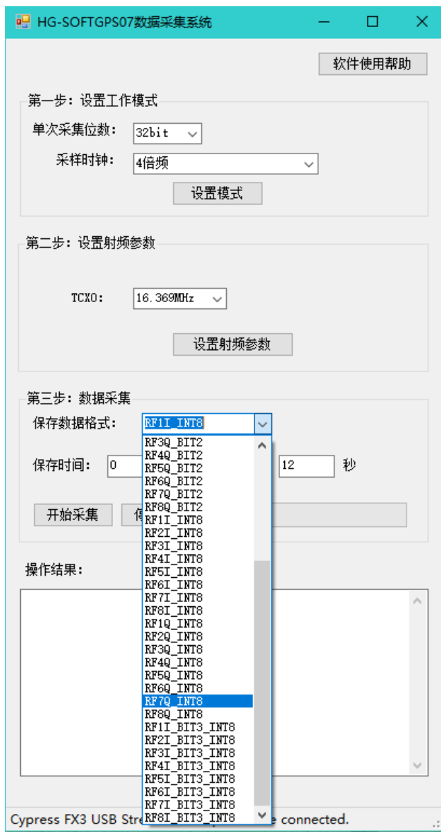
图 5 HG-SOFTGPS07 采集程序界面
