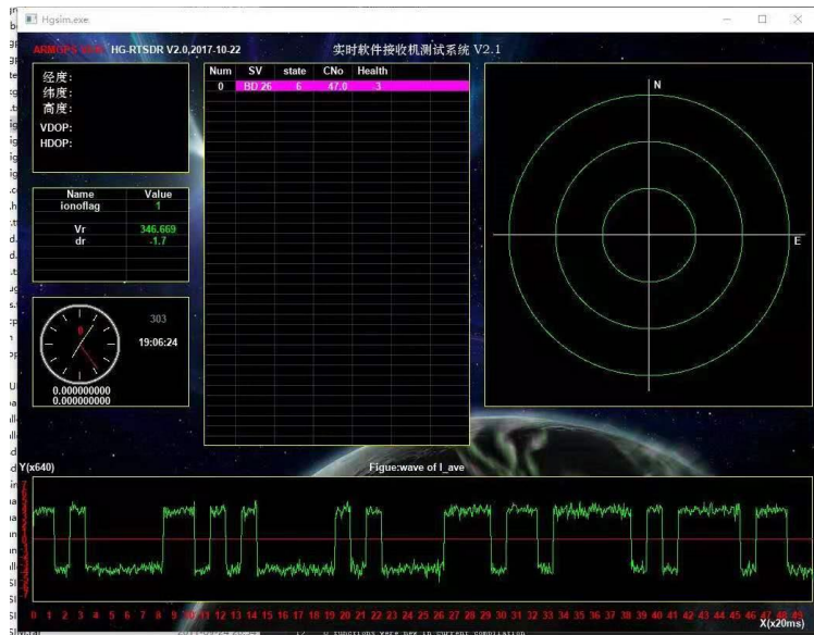
图 4 HG-SOFTGPS07 采集数据跟踪 B3I 信号效果（波形显示去除了 NH 码影响）
